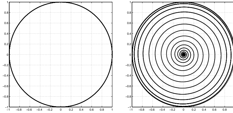
Функции \gamma_{a_1,\lambda}(x) и \gamma_{a_2,\lambda}(x) для \lambda = 1000 .
