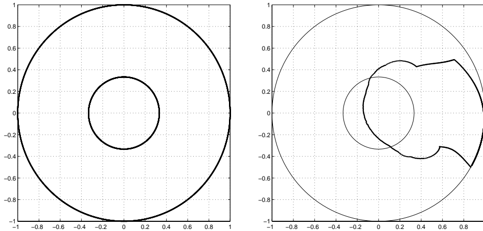
Символ a(\theta) и функция \gamma_{a,\lambda} для \lambda = 1 .
